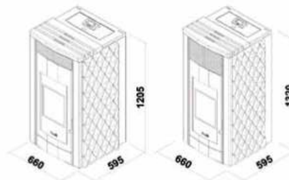
Minerva 2 Capitonè
